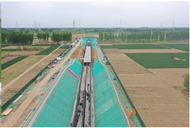
开挖面临时苫盖2021.4
