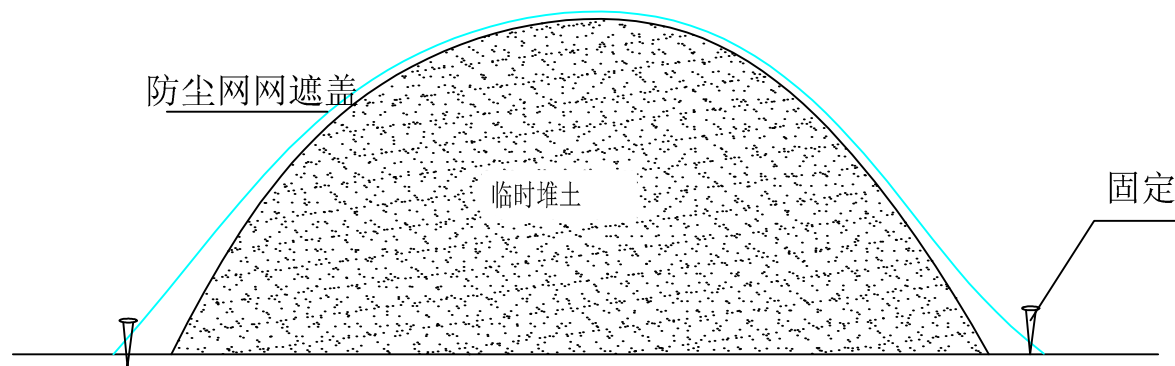
密目网遮盖设计图
